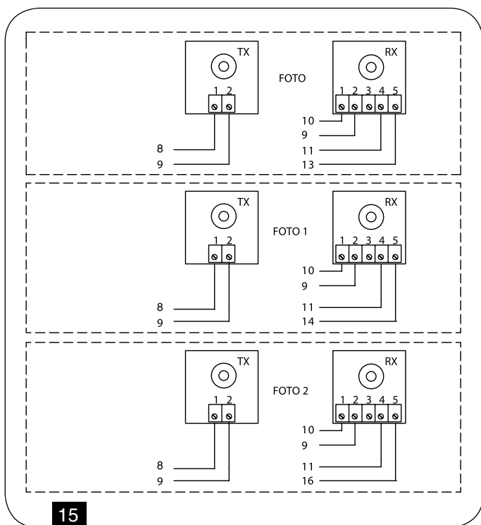
Zapojení FOTO, FOTO1 a FOTO2 (vstup AUX musí být naprogramován jako FOTO2)
