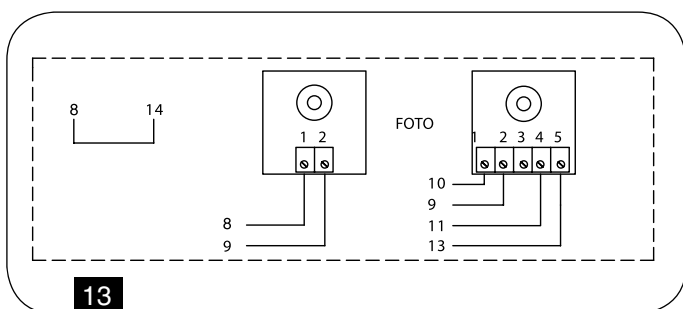
Zapojení jediného fotočlánku FOTO
