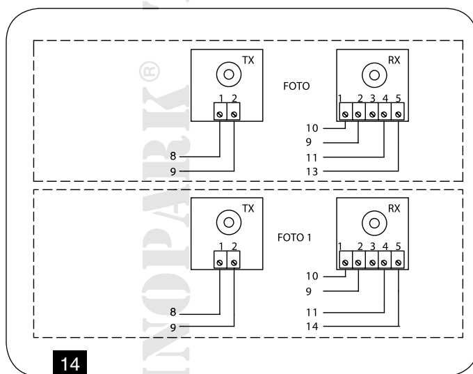
Zapojení FOTO a FOTO1
