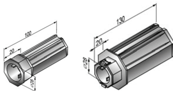
Koncovka hřídele - KU40
