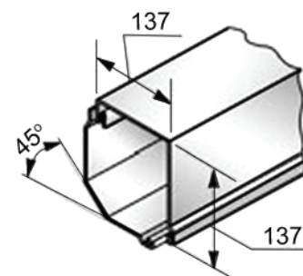
Roletová schránka - SB45/137
