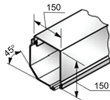
Roletová schránka - SB45/150
